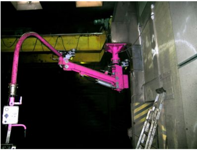
Reinigungsmanipulator
