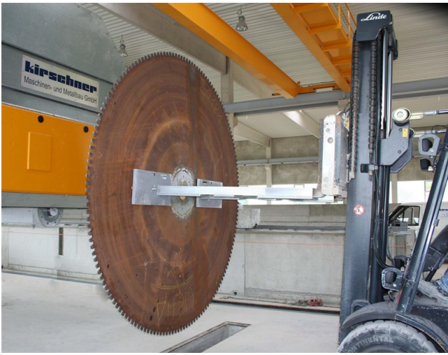
Sägeblattumsetzung
